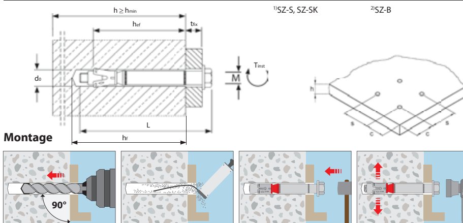
Maße Senkkopf für SZ-SK A4 [mm]
