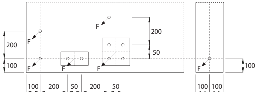
Bild 1: maximale Tragfähigkeit
