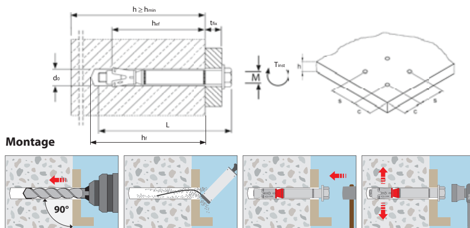
Maße Senkkopf für SZ-SK [mm]
