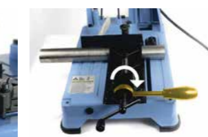
Schraubstock mit Schnellspannsystem für Serienschritte Art.Nr. 1501128
