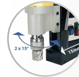
Schwenkbare Grundplatte: 2 x 15° Verschiebbare Grundplatte: 15 mm
